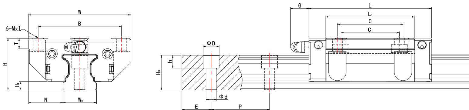
TIWINOK 品牌 12 系列高扭矩直线导轨 (俗称 KG) 法兰螺孔型滑块尺寸表
